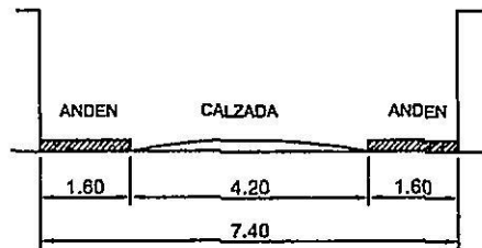
CORTE AA CALLE - 29
